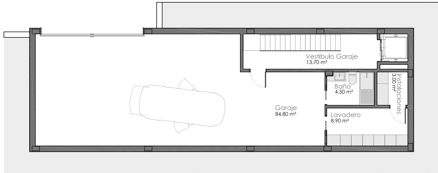
SEMISÓTANO. NIVEL -1
